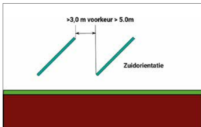
figuur 3 afstand tussen de zonnestraten
