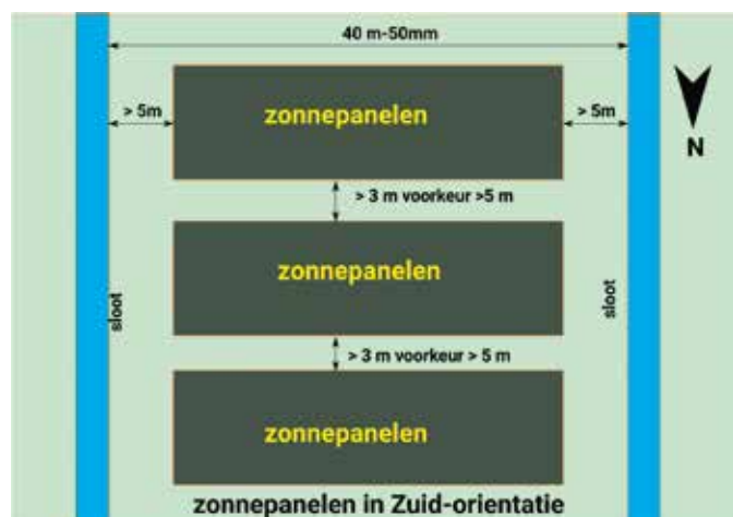
Figuur 4 voorwaarden oriëntatie en afmetingen zonneparken in de Alblasserwaard
